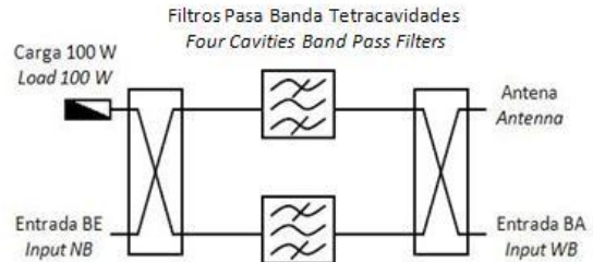
CONFIGURACIÓN DIPLEXOR CARGA CONSTANTE CONSTANT IMPEDANCE CONFIGURATION
