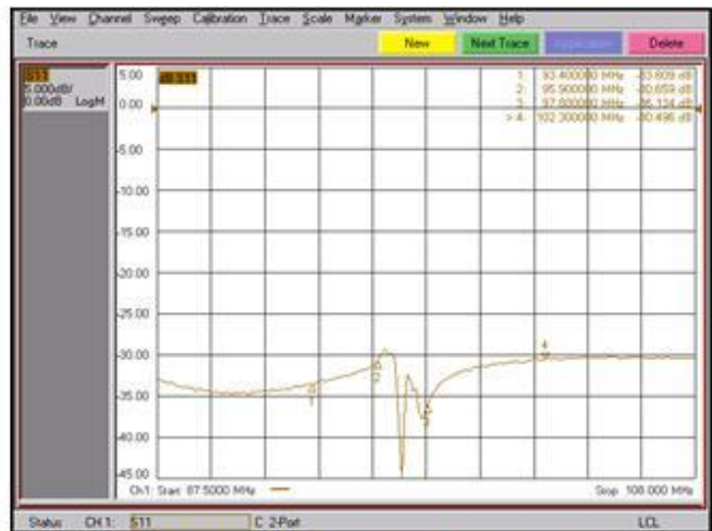
PÉRDIDAS DE RETORNO BA / RETURN LOSS WB
